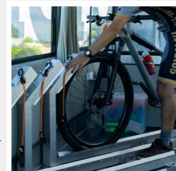
専用ラックにセットし、しっかりと溝に入れ込む ※最大タイヤ幅 64mm
